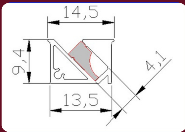
WARDROBE PROFILE W-Z1309
